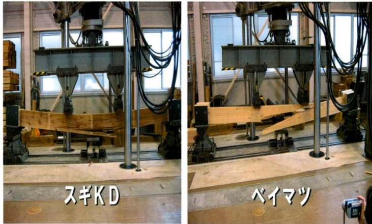
土佐材スギE70と米マツの、E110の曲げ強度は30、6ほぼ同じ。
